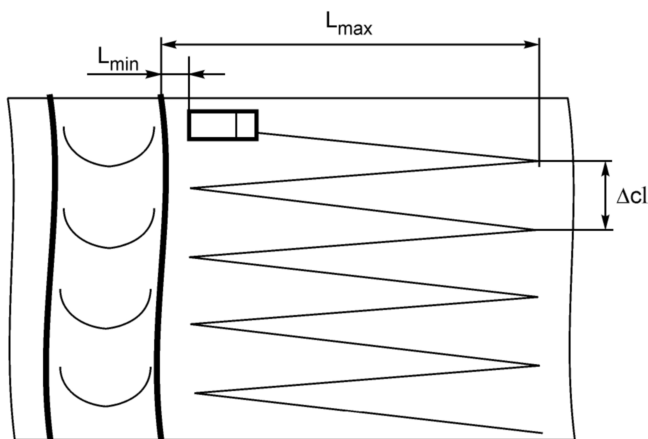
Рисунок 19 — Варианты способа поперечно-продольного сканирования
