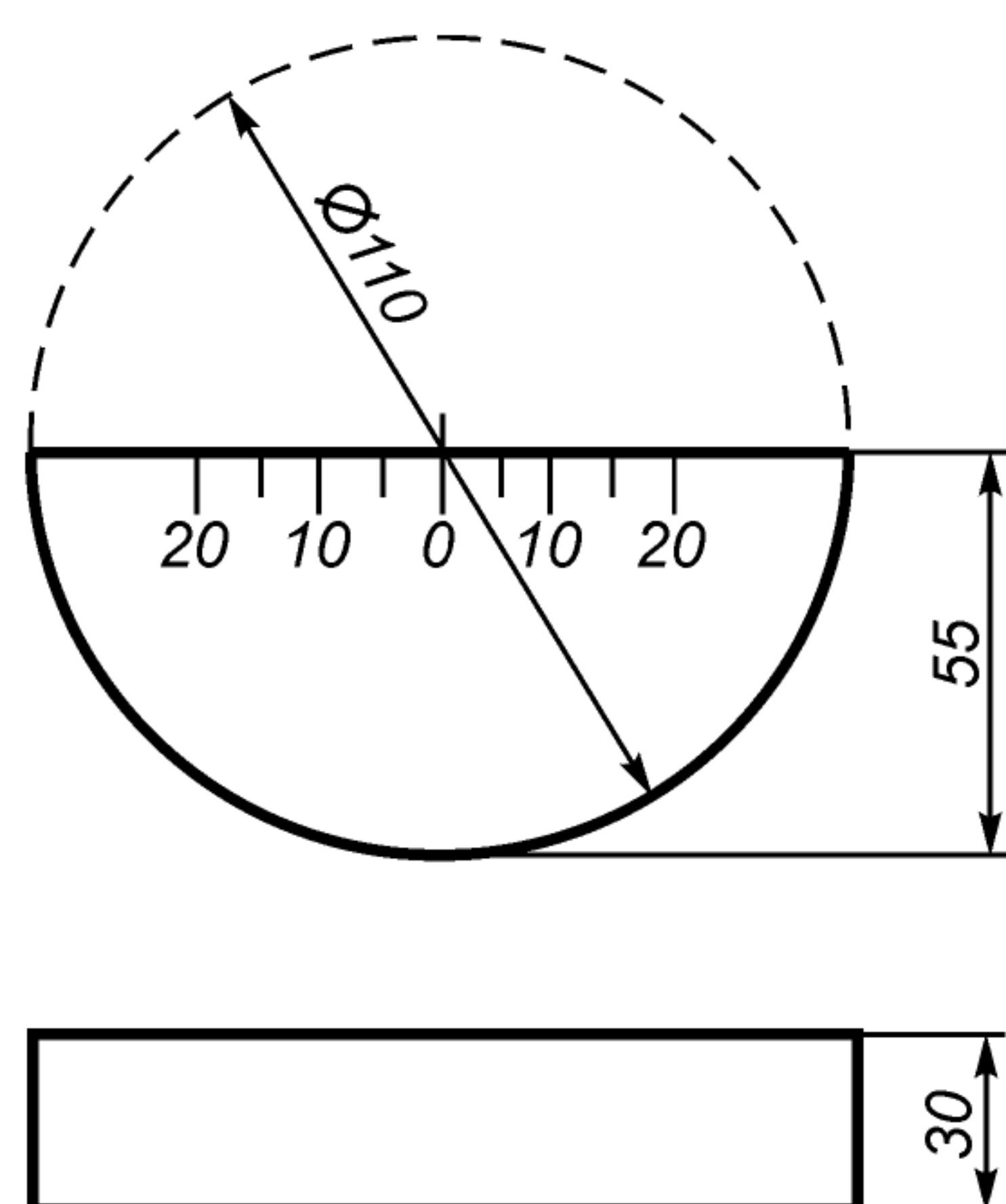
Рисунок А.2 — Эскиз меры СО-3
